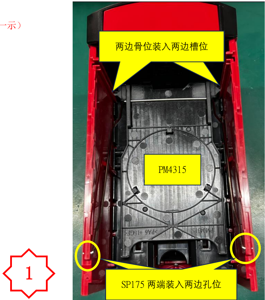
图一，将 PA3845-1 上的 PM4315 两边骨位装入 PM2625 两边槽位， 将 SP175 两端插入 PM2625 两侧孔内
