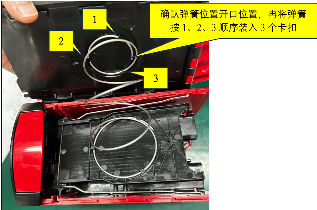
图一，将 SP2436 小圈卡入 PA4201 组件上的 PM671 槽内相应位置，按图示顺序将弹簧装入，检查大圈弹簧是否卡好。
