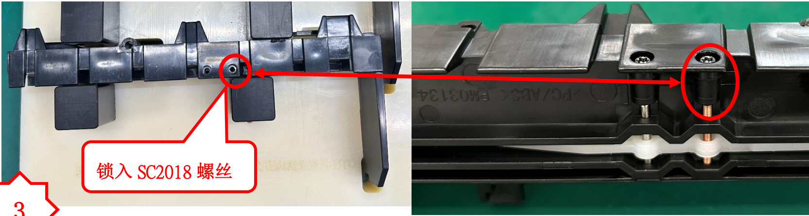
图三、将 PM3134 装好 SP2085 弹簧的组件放入治具, 锁入 SC2018 螺丝。
