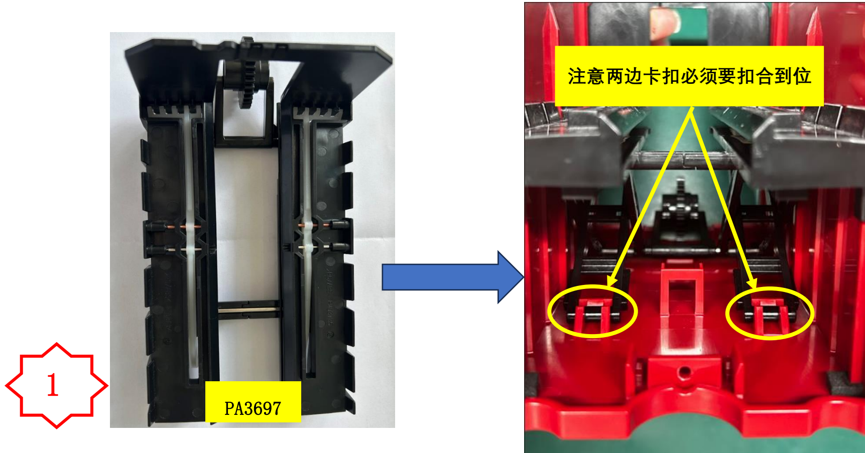
图一，将 PA3697 组件滑入 PM2625，注意两卡扣需要扣合到位，上下滑动 PA3697 组件是否顺畅。
