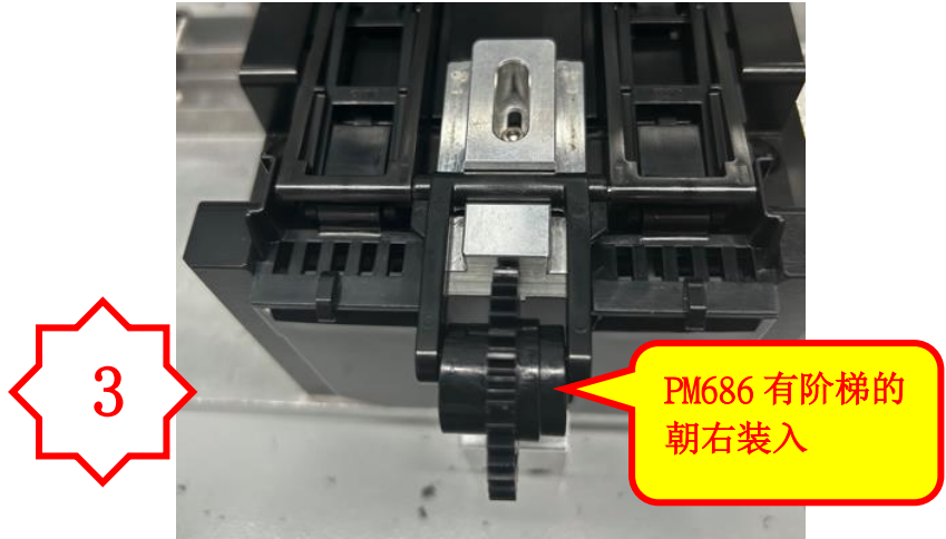
图三， 压合后将刷了油的 PM686 有阶梯的朝右装入。
