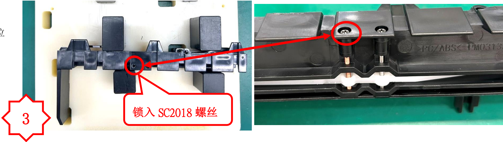
图三、将 PM3135 装好 SP2085 弹簧的组件放入治具, 锁入 SC2018 螺丝。
