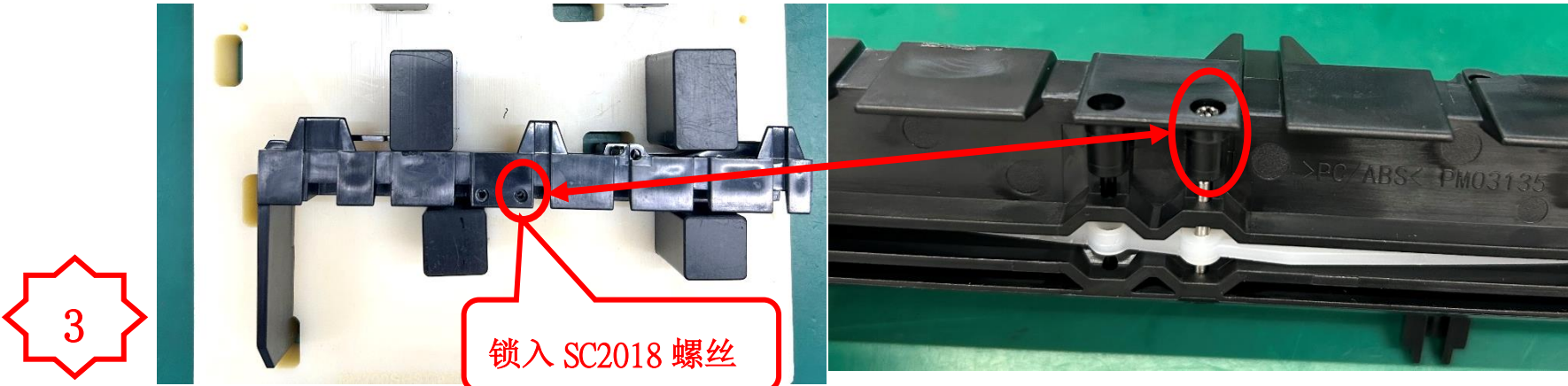
图三、将 PM3135 装好 PM3137、MC3282 的零件放入治具, 锁入 SC2018 螺丝。
