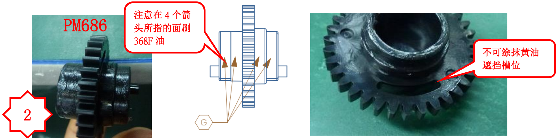
图二、在指定位置刷适量的油，检查图三位置不能有油，避免遮挡
