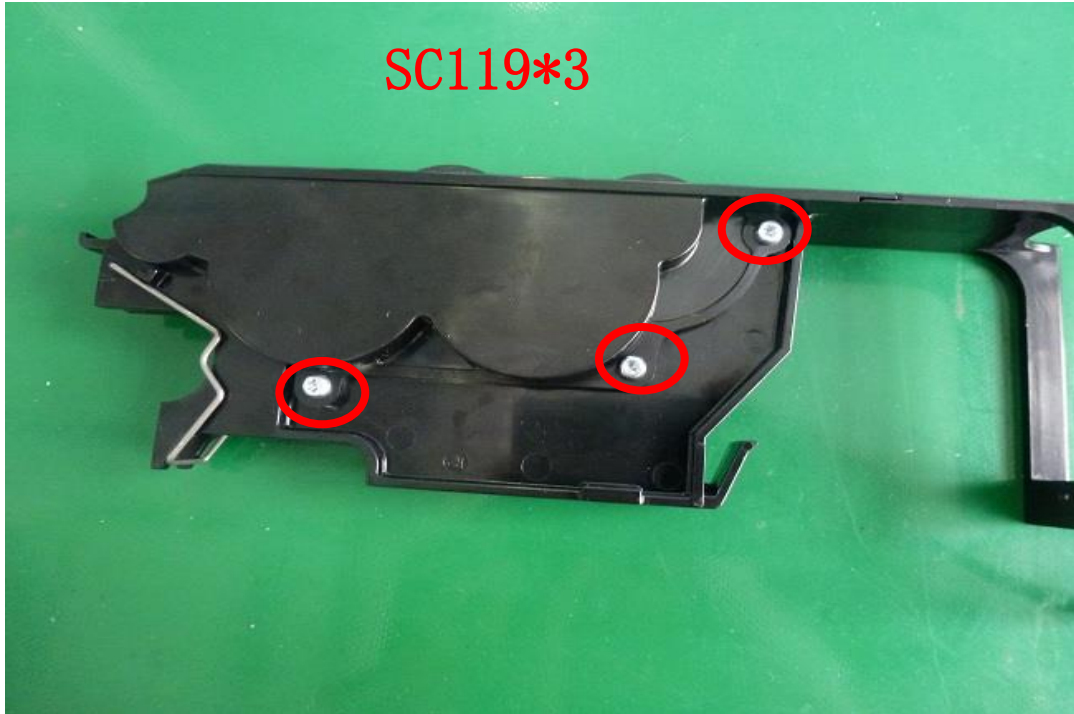
图一, 在图示位置锁上三颗 SC119 螺丝
