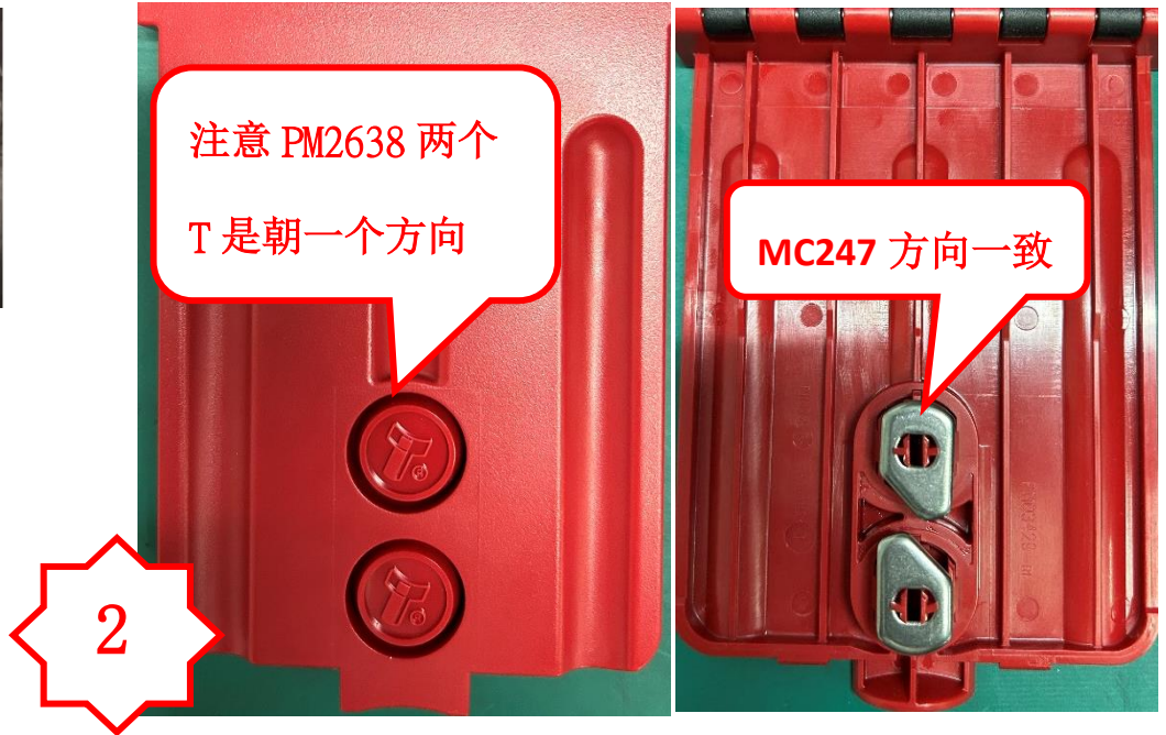
图二，检查 2 个锁的方向和 MC247 方向是否与图中方向一致
