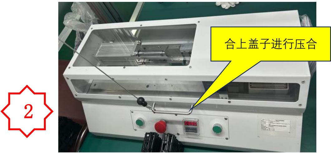
图二， 检查物料摆放 OK 后将治具盖子盖上进行压合。
