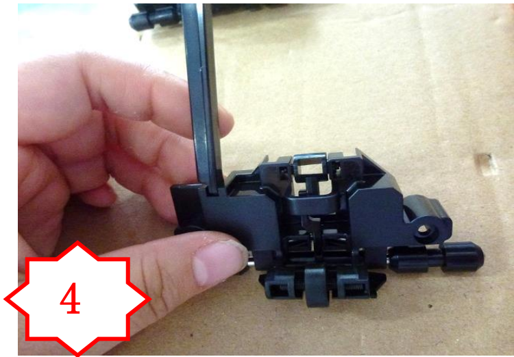
图四,将装好 SP157 的 PM683 装在 PA2742-4 中
