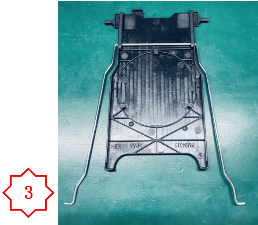
图三 ， 将 SP175 中间位置装装在 PM4315 两边的槽内
