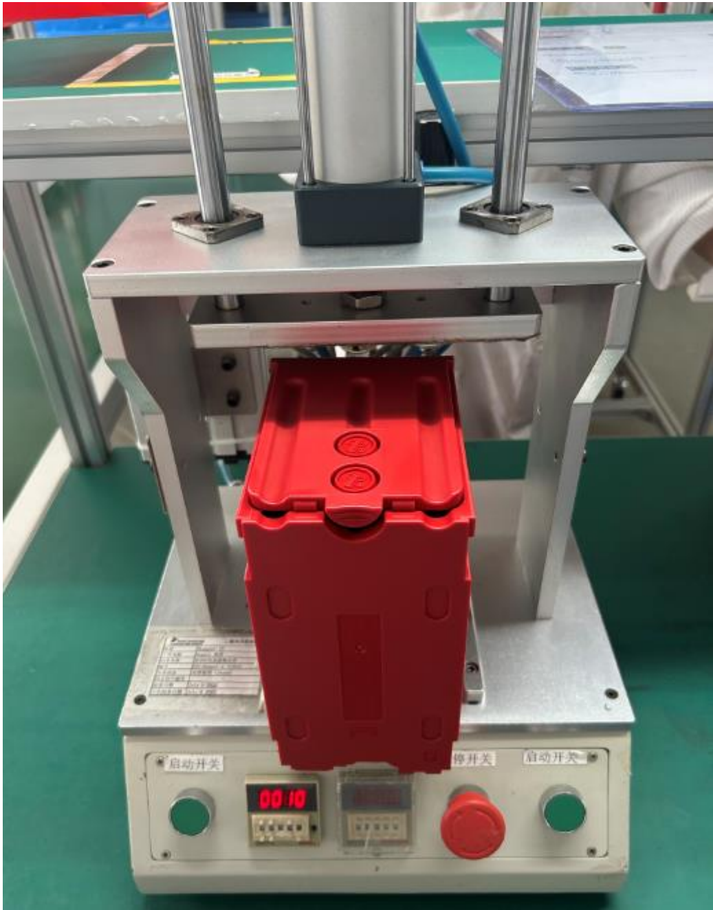
图一，将钱箱如图放入治具中，双手按住两个绿色按钮压合组件。
