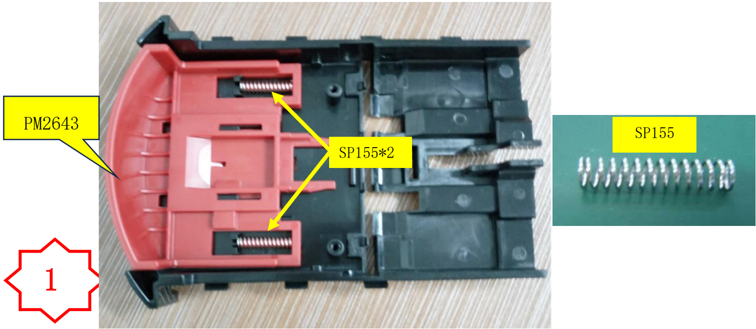
图一，装上 PM2643，并将两个 SP155 弹簧装到对应位置
