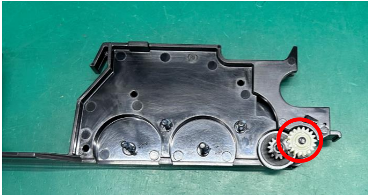
图二, 按照如片操作所示装上 PM635 齿轮
