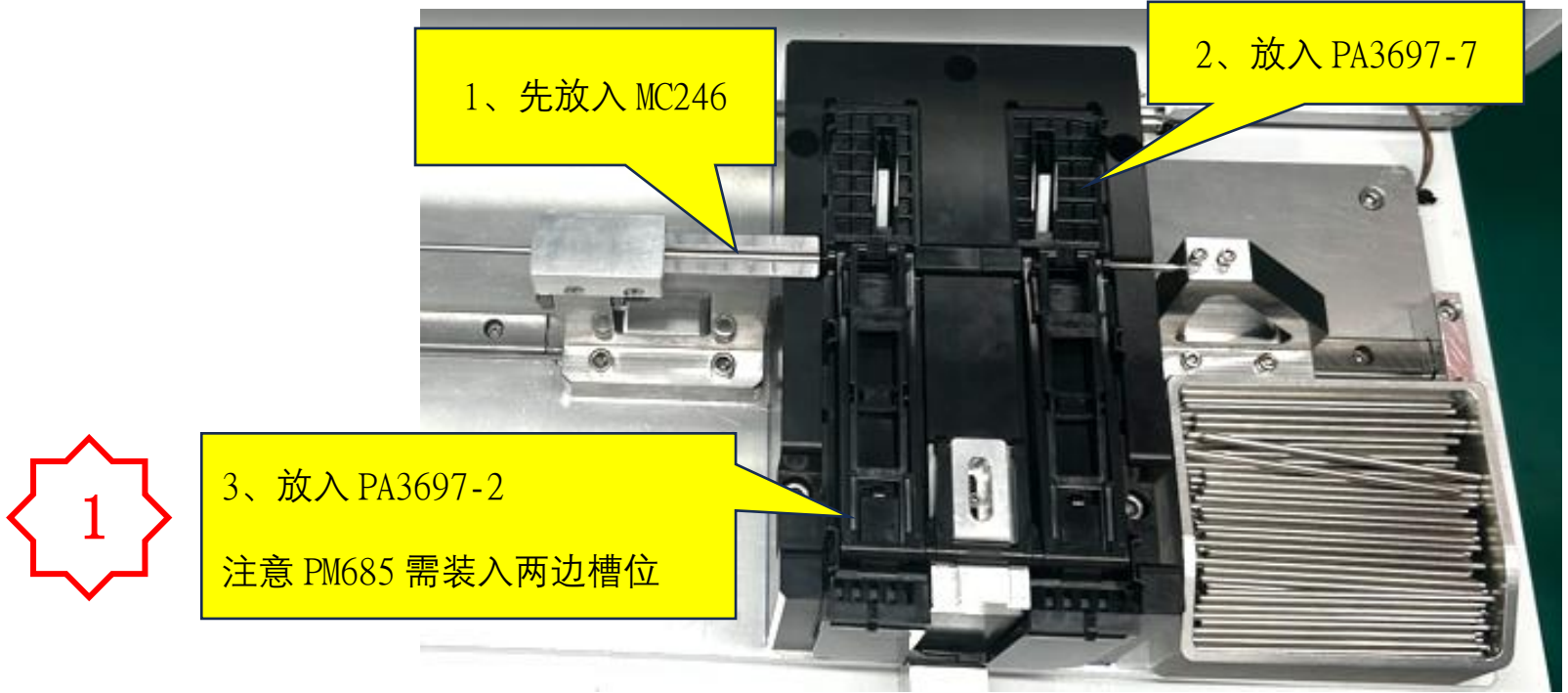
图一， 先将 MC246 放入治具槽位，再放入放入 PA3697-7 组件，最后装入 PA3697-2
