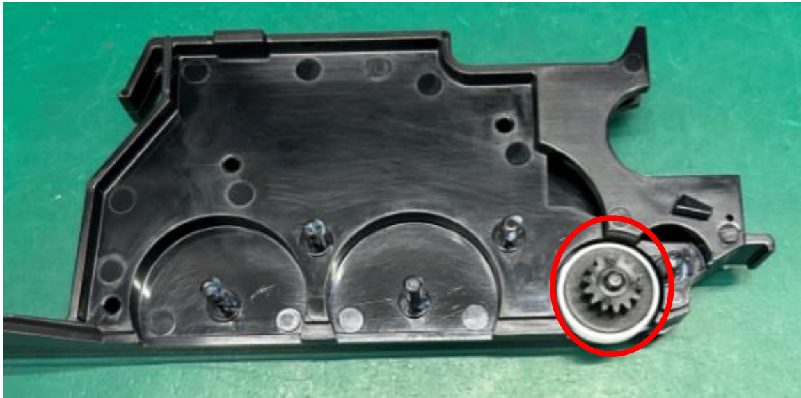
图三，按照图片操作所示，装上 PM2899
