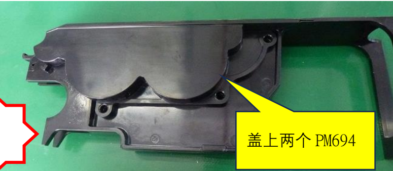
图三，按照图片操作所示，将装好齿轮的组件盖上 PM694
