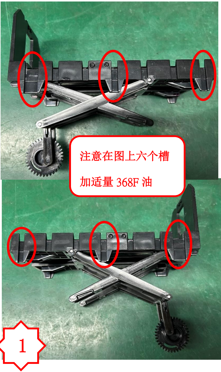
图一, 分别在 PA3697 组件两侧的三个槽内(红圈标识)刷适量的 368F 油。
