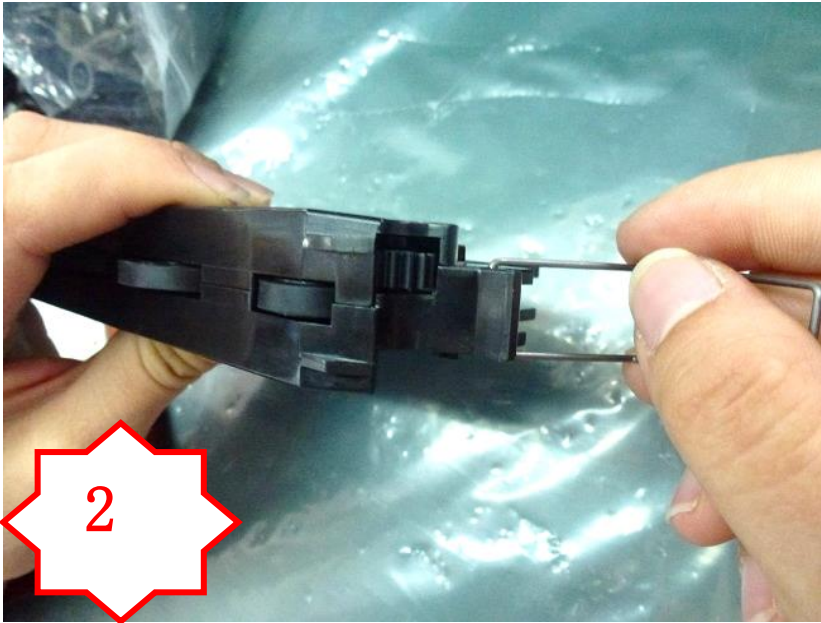
图二，将 SP204 装在 PM693 的两侧的孔内
