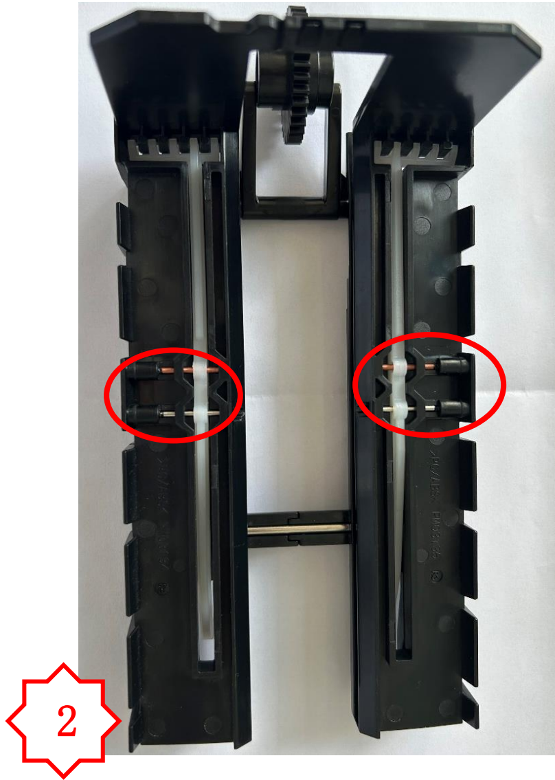
图二, 检查 SP2085\MC3282 装配位置正确, SC2018 螺丝打到位后无裂纹, 打不到位等不良, PM3136\PM3137 装配到位后回弹顺畅, 不能有卡顿现象。
