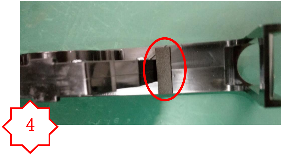
图四，将 LB2104 如图贴到 PM693 组件上。
