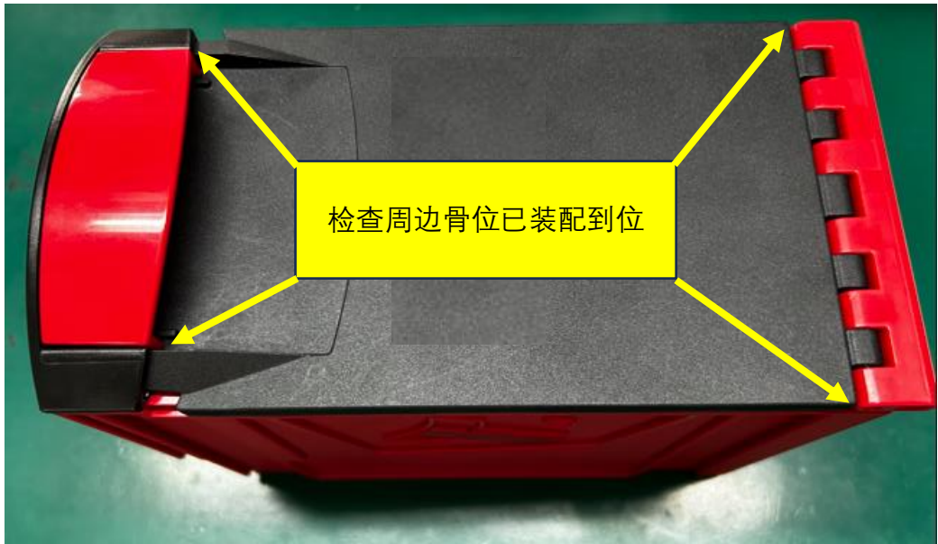
图二，PA4201 组件上的 PM671 顺着 PM2625 的槽位推到 PM2643 下等待压合
