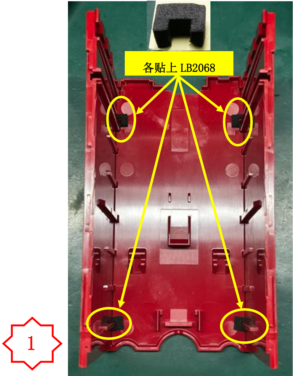
图一，在 PM2625 边上 4 个骨位分别贴上 LB2068，注意贴合位置。
