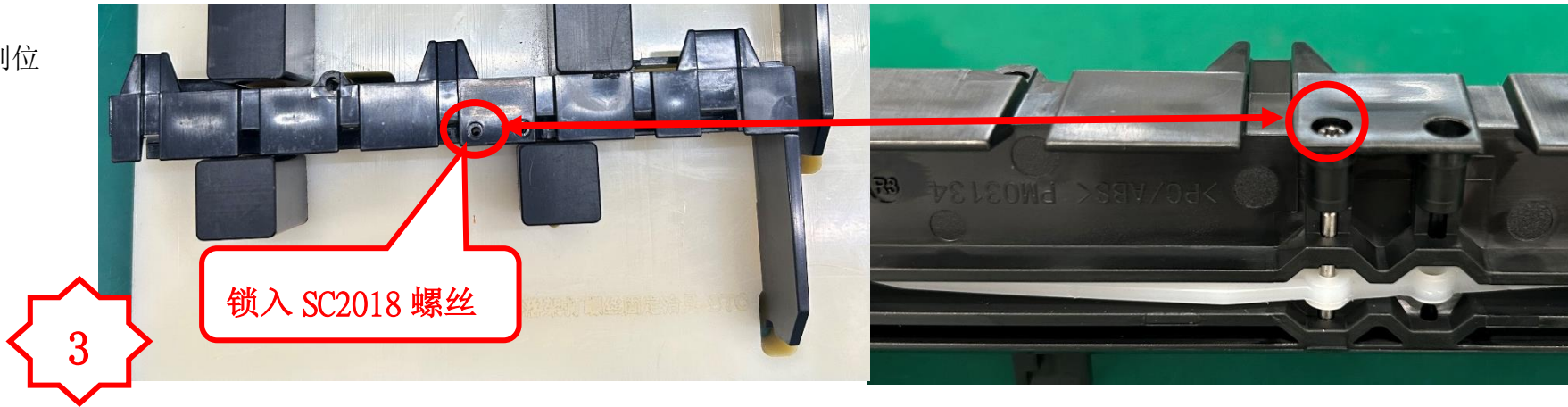
图三、将 PM3134 装好 PM3136、MC3282 的组件放入治具, 锁入 SC2018 螺丝。
