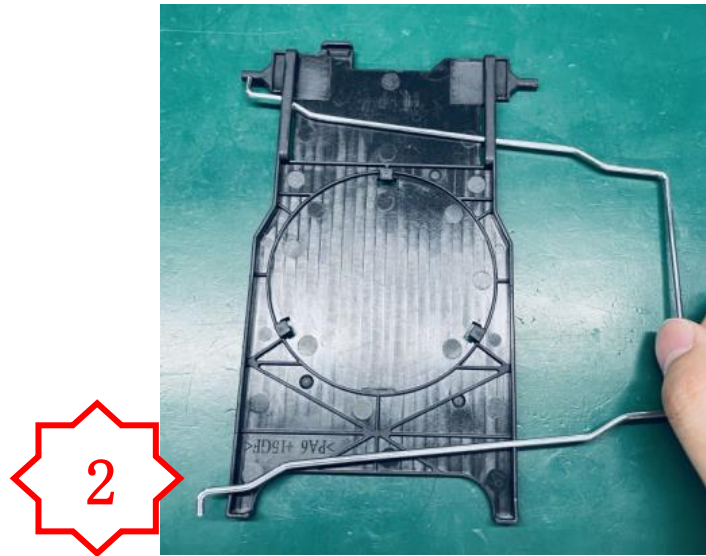
图二，将 SP175 任何一边先穿入 PM4315 的槽内
