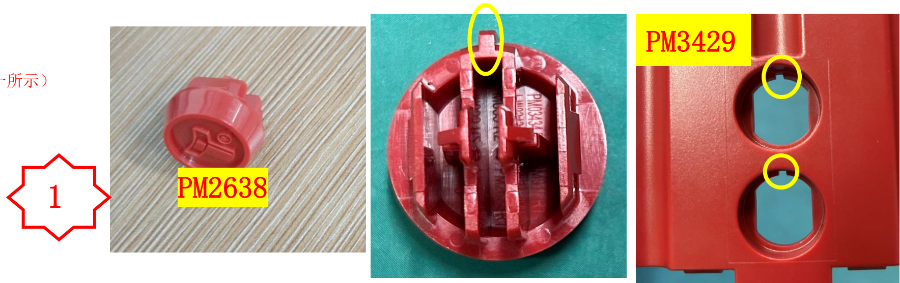
图一，将 2 个 PM2638 凸台对准 PM3429 凹槽，将卡扣扣入孔内，扣合到。
