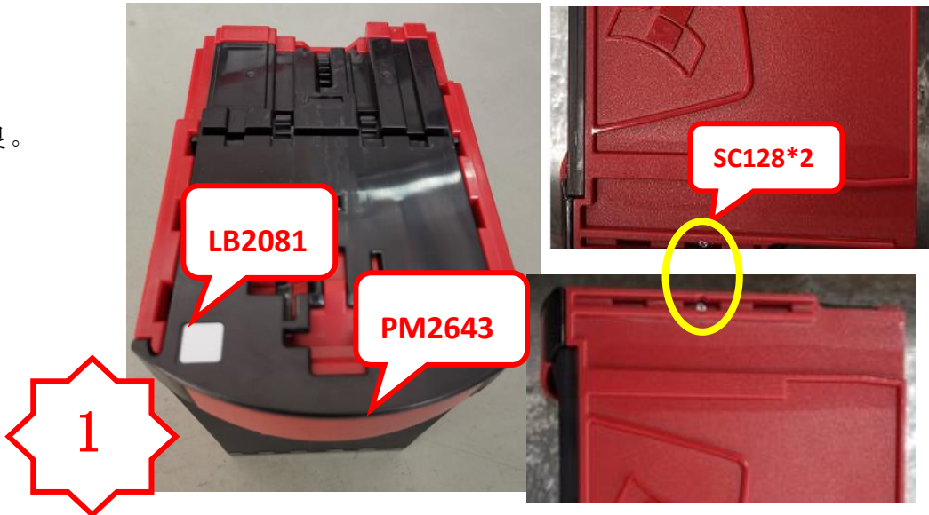
图一，拉动 PM2643,检查是否能回弹顺畅，检查 2 颗
