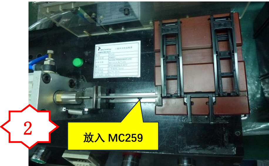
图二，将 MC259 放入治具槽位。
