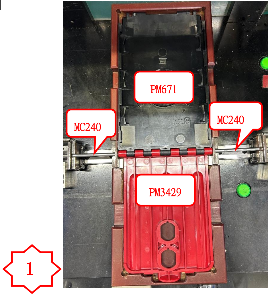
图一, 将 PM3429/PM671 装在治具如图的位置, 再在两边分别放入 MC240 (如图示)
